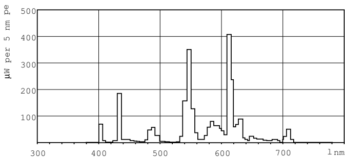
Цвет излучения /830
